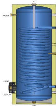
Çift Sıra Serpantinli Isı Pompası Boyleri
