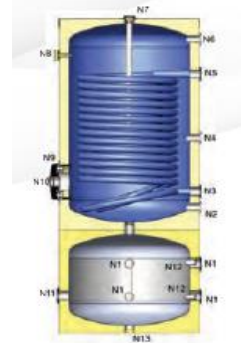
Kompakt ( Isı Pompası Boyleri + Buffer ) Boyleri
